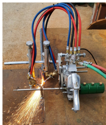
BA 200-2T on Edge Tracing Guide
